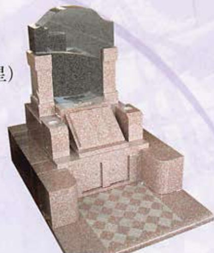
No.48 石種：G654(南星) 才数：59.337 才 幅：188cm 奥行：249cm 高さ：217cm
